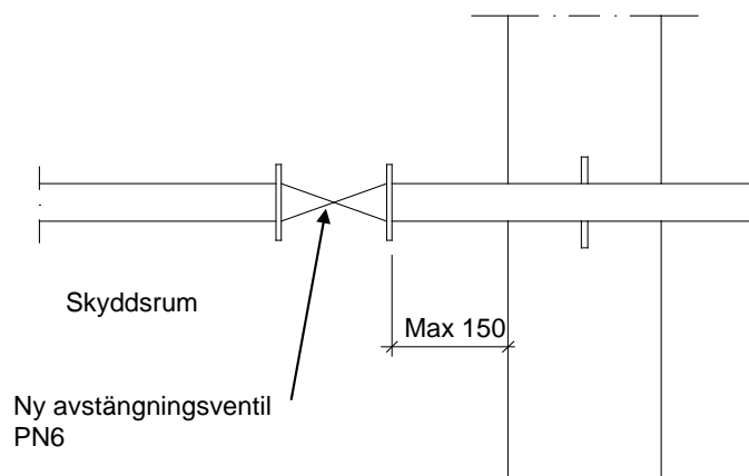
Figur T17-107a. Vy av avstängningsventil.
